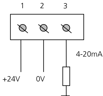
Abb. 2: Anschlußbelegung MF420-P.
